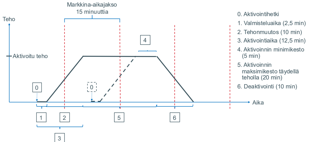
Kuva 222 Suoran aktivoinnin periaate 12,5 min aktivointiajalla
