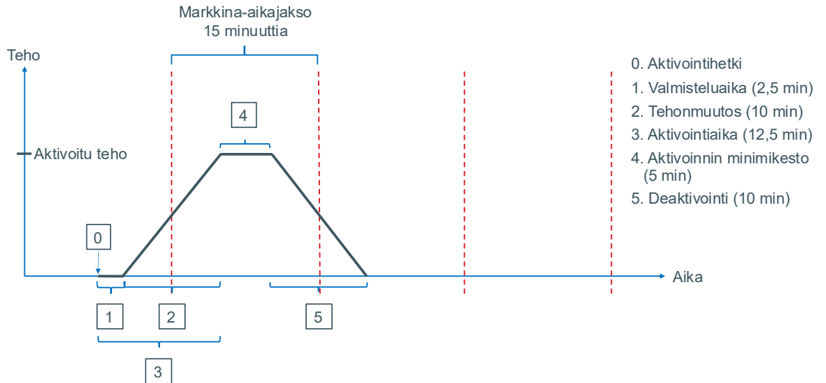
Kuva 114 Ajastetun aktivoinnin periaate 12,5 min aktivointiajalla
