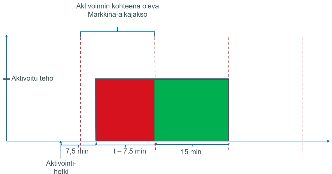
Kuva 121242 Esimerkki Suoran aktivoinnin energiamaksun perusteena olevasta energiasta
