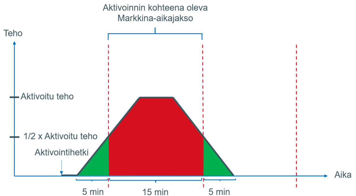
Kuva 333 Ajastetun aktivoinnin Aktivoidut säätö energiamäärät eri Taseselvitysjaksoille
