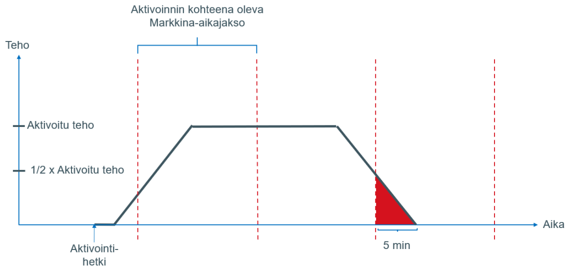
Kuva 111144 Suoran aktivoinnin kohteena olevaa Markkina-aikajaksoa seuraavaa Markkina-aikajaksoa seuraavalle Taseselvitysjaksolle kohdistuva Aktivoitu säätöenergia
