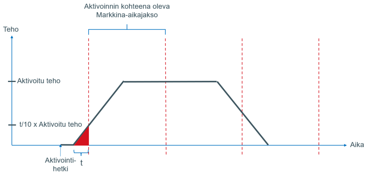
Kuva 444 Suoran aktivoinnin kohteena olevaa Markkina-aikajaksoa edeltävälle Taseselvitysjaksolle kohdistuva Akti- voitu säätö energia, kun Tehonmuutos alkaa ennen Suoran aktivoinnin kohteena olevaa Markkina-aikajaksoa
