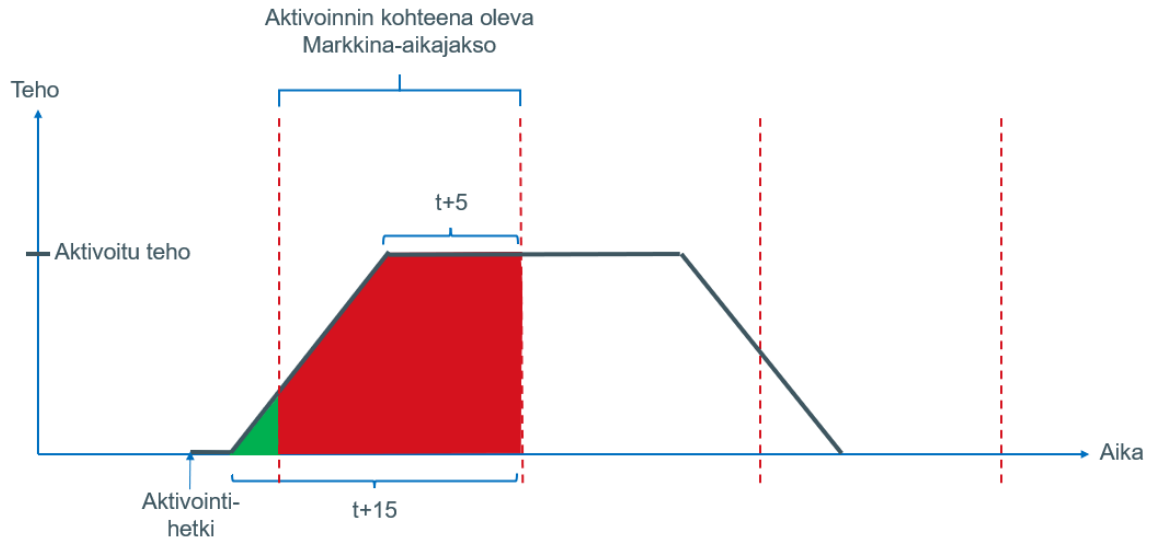
Kuva 666 Suoran aktivoinnin kohteena olevaa Markkina-aikajaksoa vastaavalle Taseselvitysjaksolle kohdistuva Aktivoitu säätöenergia , kun Tehonmuutos alkaa ennen Suoran aktivoinnin Markkina-aikajaksoa
