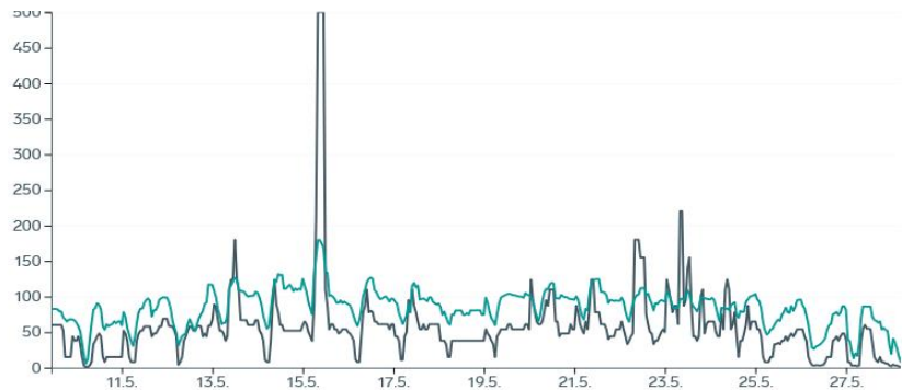
Taajuusohjattu häiriöreservi
