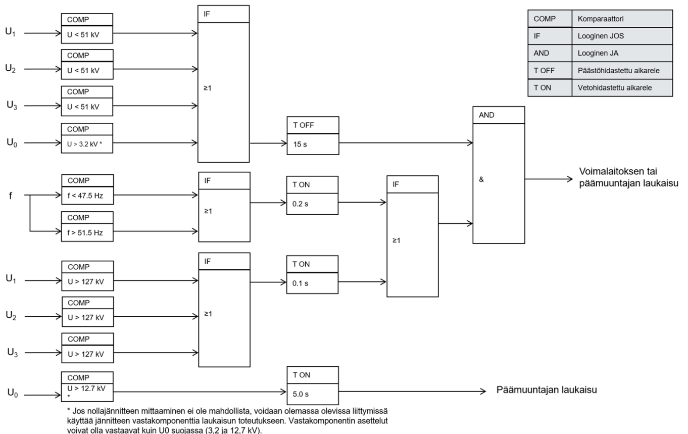
Kaavio 1. Paikallisen eroonkytkennän logiikkakaavio. Vastakomponenttijännitteen asettelussa käytetään keskijänniteverkon vaihejännitettä.
