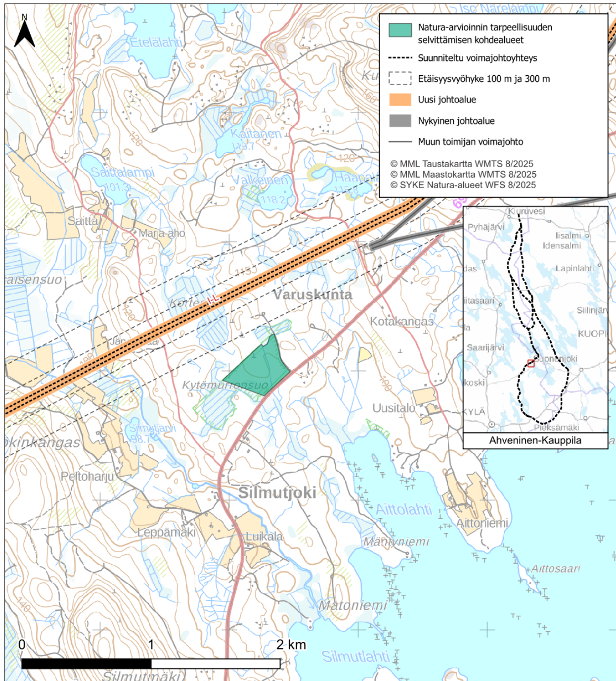
Kuva 5.1. Voimajohtoreittivaihtoehtojen sijoittuminen suhteessa Kytömurronsuon Natura-alueeseen.
