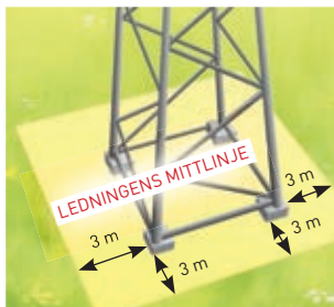
Ostagad enkelstolpe
