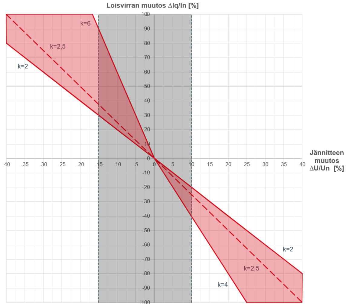
Kuva 18.5. Loisvirran aktivoitirajat jännitteen perusteella sekä k-kertoimen määrittely. Loisvirran syöttö aktivoituu harmaan alueen ulkopuolella. Nuolen alkupiste kuvaa loisvirransyötön aktivoitumista ja suunta lisäloisvirran kasvua jännitepoikkeaman kasvaessa. Punainen alue kuvaa DFIGN-voimalaitoksen k-kertoimen asettelualuetta. Katkoviiva kuvaa täyssuuntaajalaitoksen kulmakerrointa k = 2,5 .
