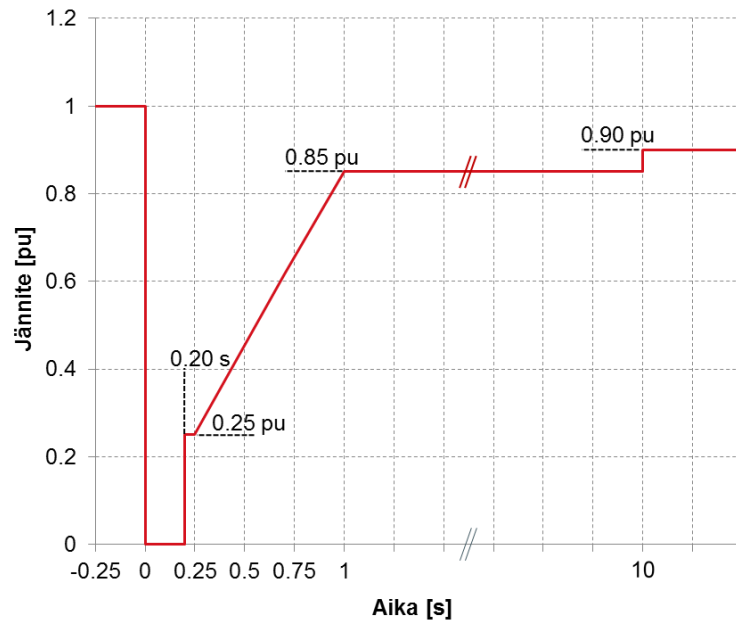
Kuva 10.9. Lyhytaikaista jännitehäiriötä vastaava liittämispisteen jännite, jonka aikana ja jälkeen tyyppin D tahtikonevoimalaitoksen, jonka liittämispisteen nimellisjännite on vähintään 400 kV, tulee jatkaa toimintaansa normaalisti. Jännitteen suhteellisarvo 1,0 pu on jännite ennen häiriötä. Jännite on 0,00 pu 200 millisekunnin ajan.
