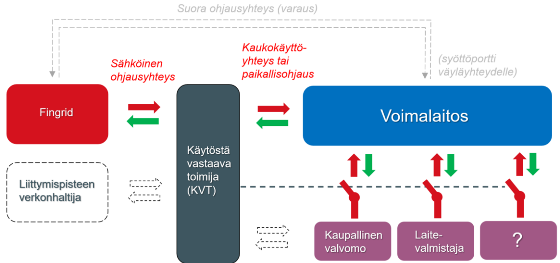
Kuva 10.4. Voimalaitoksen ohjaus ja kaukokäyttö. Voimalaitoksen käytöstä vastaava toimija operoi voimalaitosta. Fingrid voi antaa voimalaitokselle ohjauksia (punaiset nuolet) sekä vastaanottaa tilatietoja (vihreät nuolet) sähköisellä ohjausyhteydellä. Erillisen, suoran Fingridin ja voimalaitoksen välisen ohjausyhteyden toteuttamisesta päätetään erikseen. Käytöstä vastaavalla toimijalla voi lisäksi olla sähköinen ohjausyhteys (katkoviivanuolet ylhäällä) tai muuta tiedonvaihtoa mahdollisen liittymispisteen verkonhaltijan (esim. jakeluverkkoyhtiö) tai muiden voimalaitosta mahdollisesti ohjaamaan kykenevien toimijoiden kanssa (katkoviivanuolet alhaalla). Käytöstä vastaavalla toimijalla on mahdollisuus oikeuttaa ja rajoittaa muiden toimijoiden ohjauskykyä.
