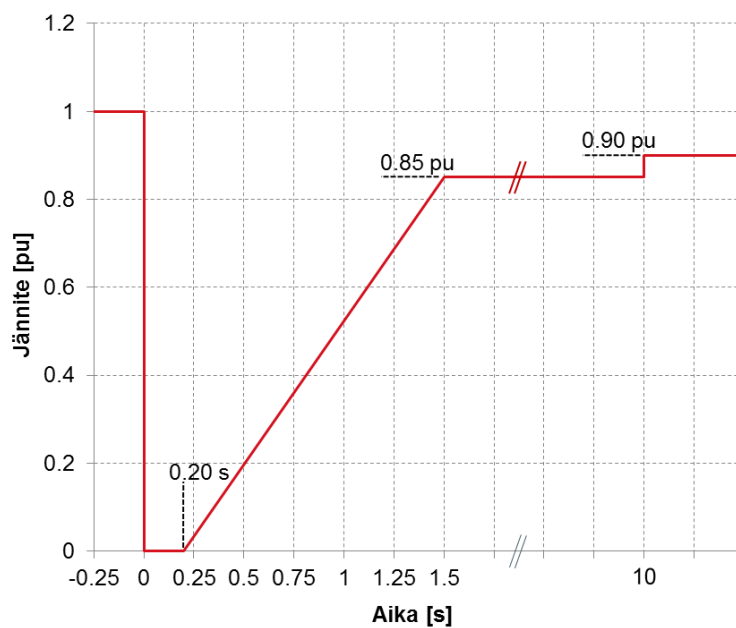
Kuva 10.10. Lyhytaikaista jännitehäiriötä vastaava liittämispisteen jännite, jonka aikana ja jälkeen tyyppin D suuntaajakytketyn voimalaitoksen tulee jatkaa toimintaansa normaalisti. Jännitteen suhteellisarvo 1,0 pu on jännite ennen häiriötä. Jännite on 0,00 pu 200 millisekunnin ajan.
