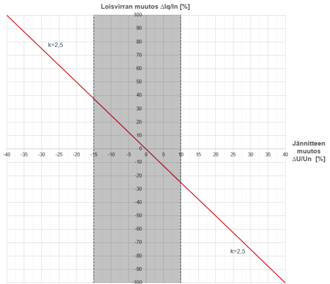
Kuva 10.3. Loisvirran aktivointirajat jännitteen perusteella sekä k-kertoimen määrittely. Loisvirran syöttö aktivoituu harmaan alueen ulkopuolella. Suora kuvaa kulmakerrointa k=2,5 .
