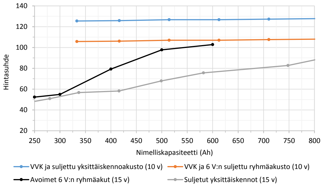
Kuva 22. Kokonaiskustannuksiltaan pienimpien ja suurimpien akustoratkaisujen sekä yhdistettyjen varavoimaratkaisujen kokonaiskustannusten netto nykyarvot, kun varavoimakonetta koekäytetään 12 kertaa vuodessa.
