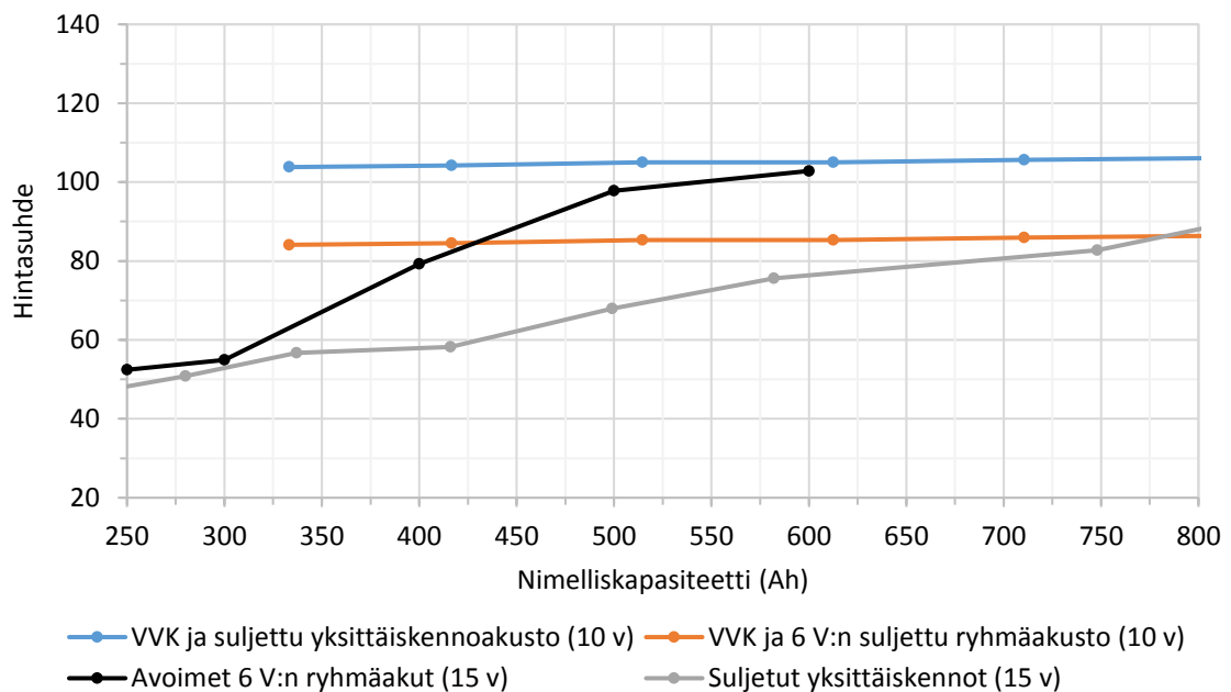
Kuva 21. Kokonaiskustannuksiltaan pienimpien ja suurimpien akustoratkaisujen sekä yhdistettyjen varavoimaratkaisujen kokonaiskustannusten nettonykyarvot, kun varavoimakonetta koekäytetään 6 kertaa vuodessa.
