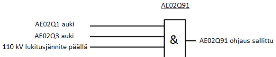
Kuva 3 Esimerkki maadoituskytkimen lukituskaaviosta [12].
