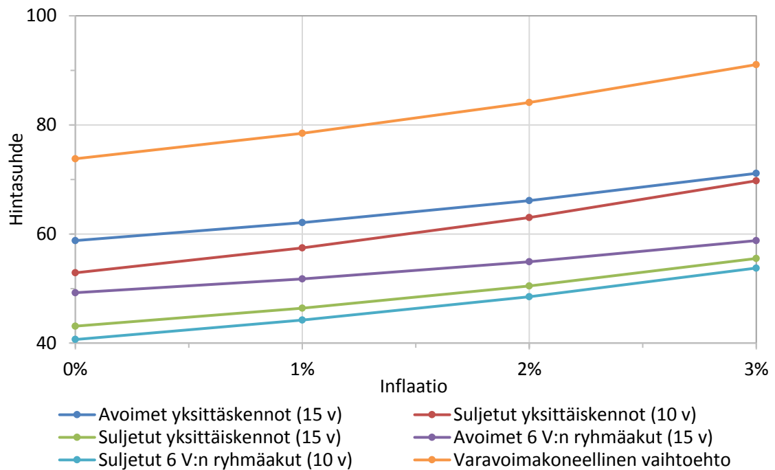
Kuva 24. Inflaation vaikutus kustannuksiin diskonttokoron ollessa 6 %.
