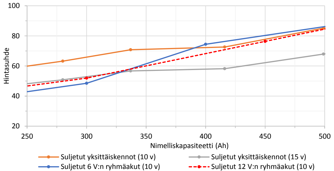
Kuva 16. Suljettujen akustojen kokonaiskustannusten nettohyönteisarvot.
