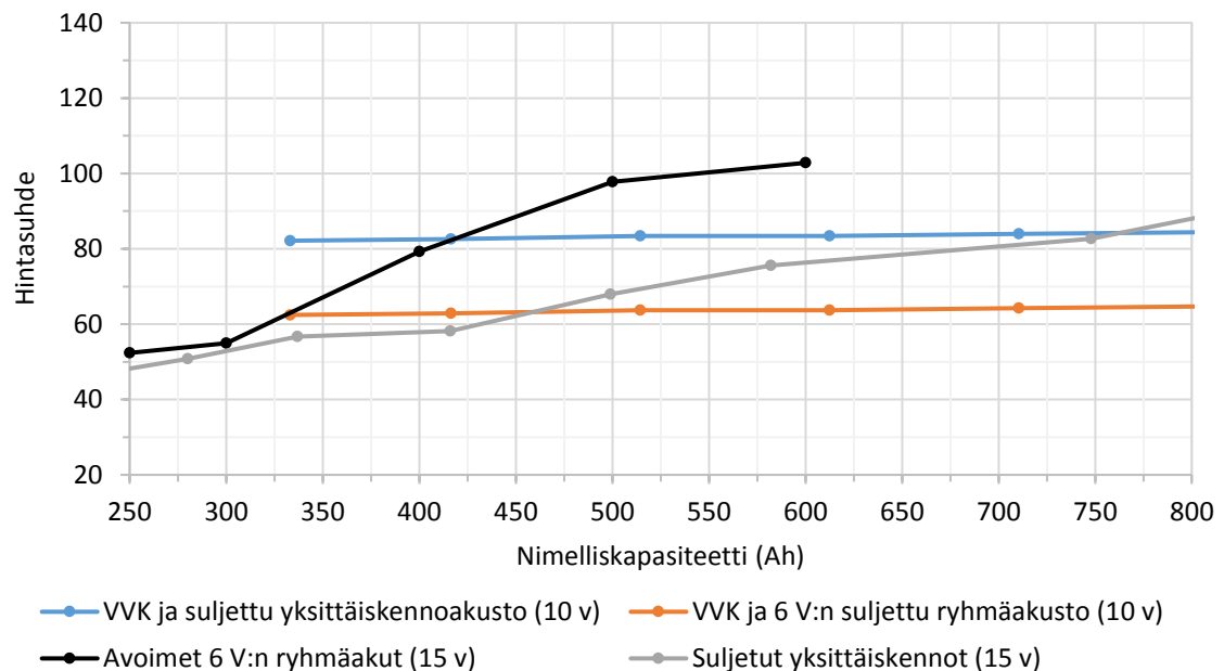
Kuva 25. Kokonaiskustannuksiltaan pienimpien ja suurimpien akustoratkaisujen sekä yhdistettyjen varavoimaratkaisujen kokonaiskustannusten nettonykyarvot, kun varavoimakoneen kaikki koe-käytöt suoritetaan kauko-ohjauksella etänä.
