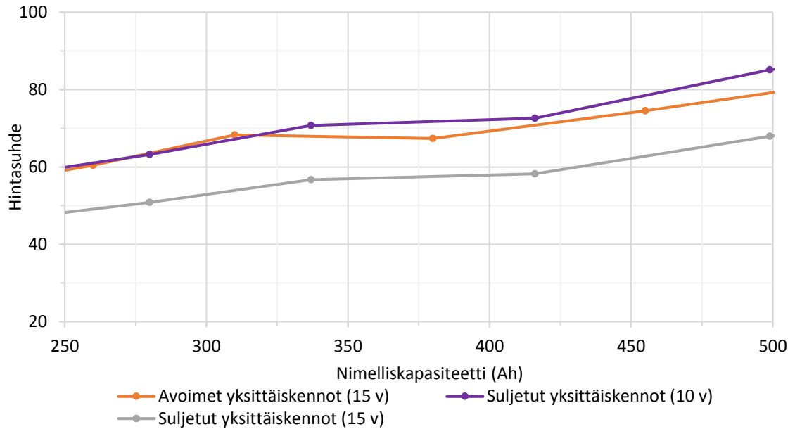
Kuva 12. Yksittäiskennoakustojen kokonaiskustannusten nettonykyarvot.
