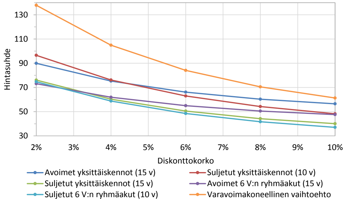
Kuva 23. Diskonttokoron vaikutus kustannuksiin inflaation ollessa 2 %.
