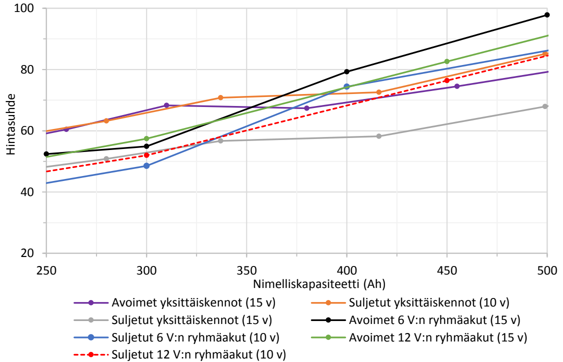
Kuva 17. Kaikkien vertailtujen akustojen kokonaiskustannusten nettohyötyarvot.
