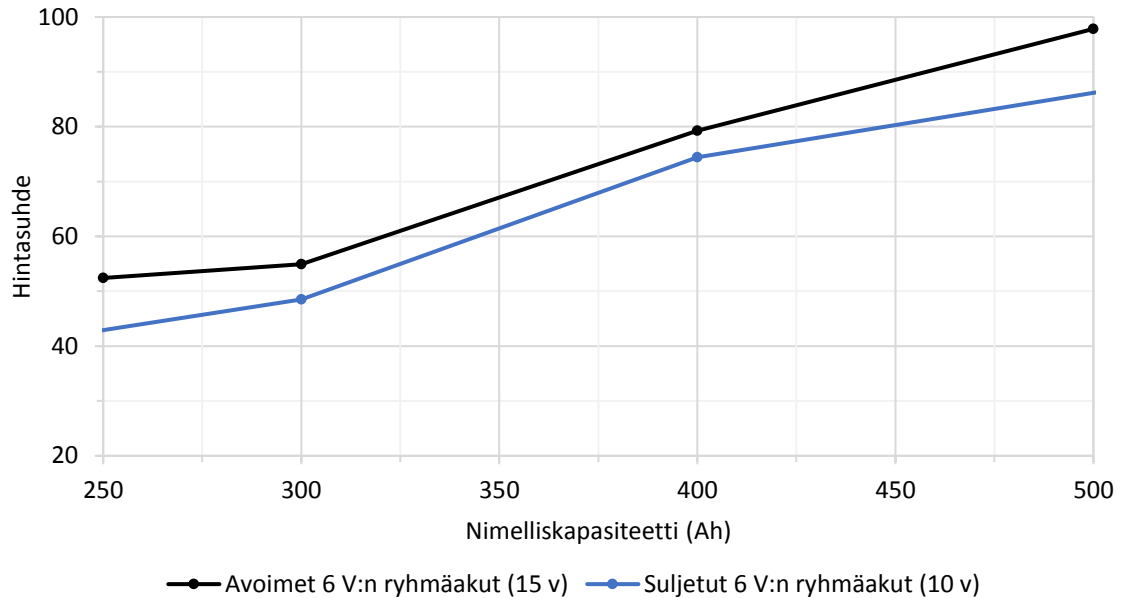
Kuva 13. 6V:n ryhmäakustojen kokonaiskustannusten nettohyödyt.
