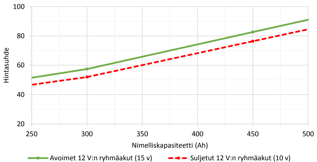
Kuva 14. 12 V:n ryhmäakustojen kokonaiskustannusten nettohyödyt.
