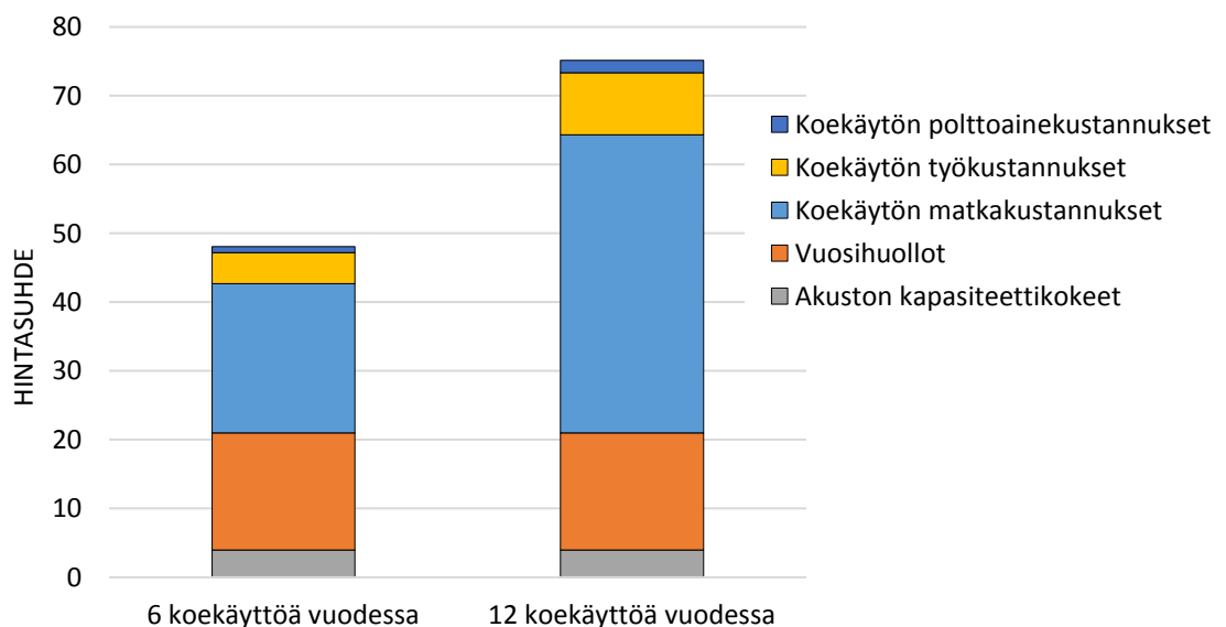
Kuva 19. Varavoimakoneellisen ratkaisun kunnossapidon kustannuslajit 6 ja 12 koekäytöllä vuodessa, kun käytettiin 20 kVA:n varavoimakonetta ja 6 V:n suljettuja ryhmäakustoa 220 V:n järjestelmässä.
