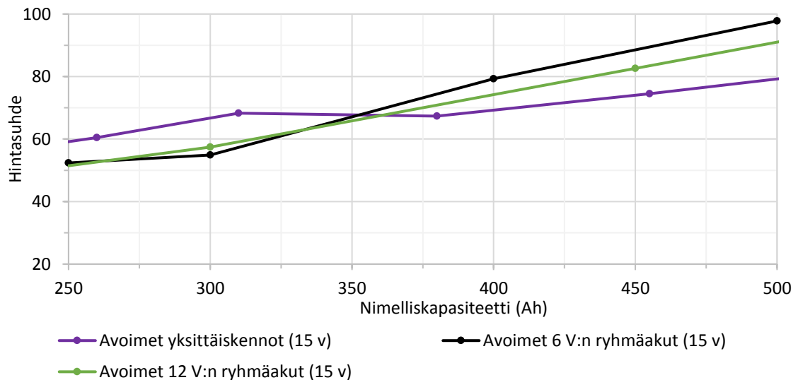
Kuva 15. Avoimien akustojen kokonaiskustannusten nettohyötyarvot.
