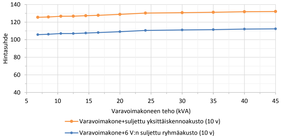
Kuva 20. Varavoimakoneellisen ratkaisun kokonaiskustannusten nettohyötyarvot eri akustoilla 220 V:n järjestelmässä.
